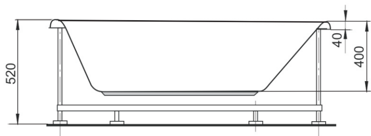
Presek "A-A"
